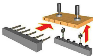
СХЕМА СБОРКИ ГОТОВОГО ИЗДЕЛИЯ
